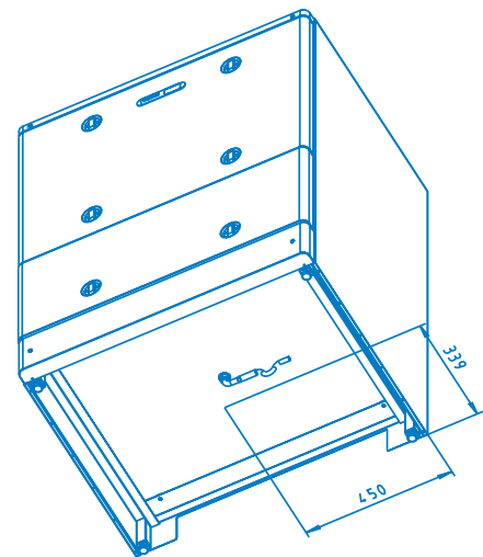
Lage des Kondenswasseranschlusses
